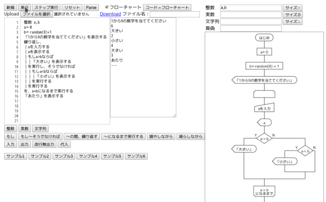
図 3 WaPEN の実行画面 Fig. 3 Snapshot of WaPEN
